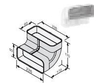
Flachkanalbogen DFK-BV 90
