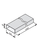
Flachkanal DFK-R 1000
