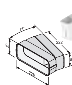
Flachkanalbogen DFK-BH 15
