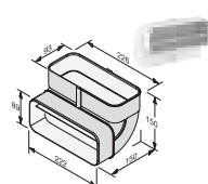
Flachkanalbogen DFK-BVK 90
