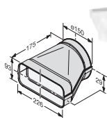
Flachkanaladapter DFK-A
