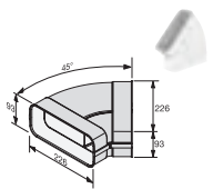
Flachkanalbogen DFK-BH 45
