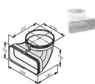
Flachkanaladapter DFK-AK 90
