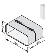
Längenausgleich DFK-L
